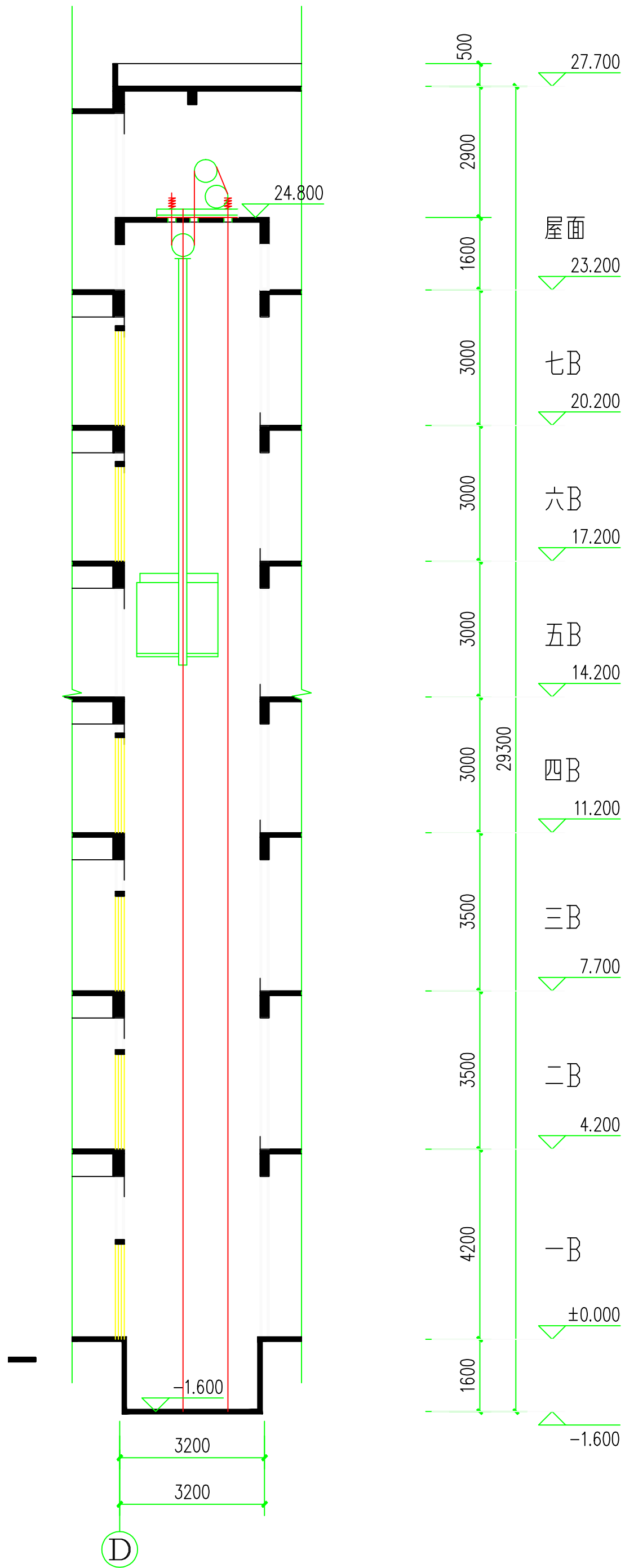
电梯局部剖面图 1:100
